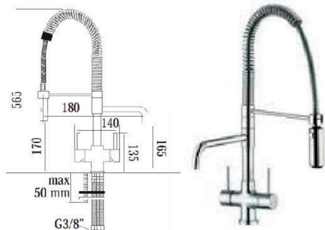
SCHÉMA DU ROBINET DOUCHETTE - MITIGEUR 3 VOIES
